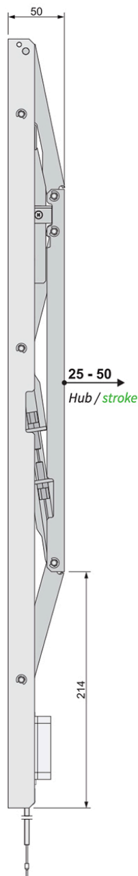
Boltekurve strammes (Aktiveret)
