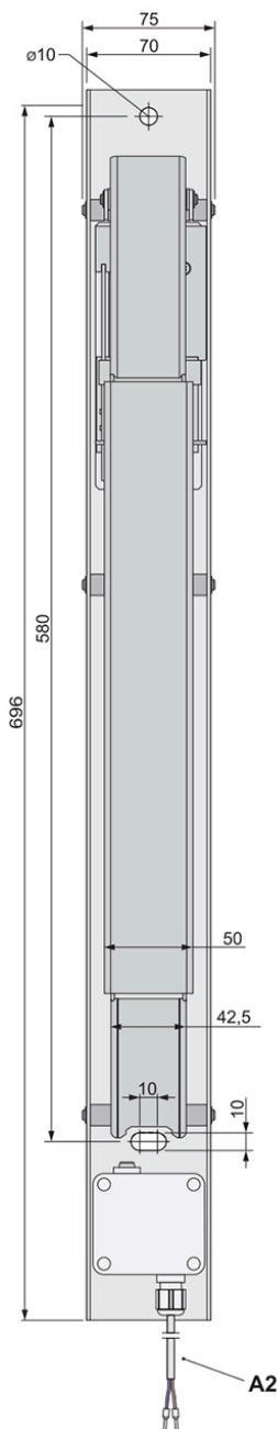
Boltekurve med motordrev og strømforsyning til 100 - 250 V AC/DC
