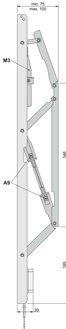
Boltekurve faldt (Frakoblet)
