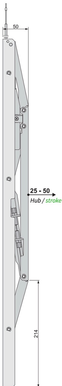
Boltekurve strammes (Aktiveret)
