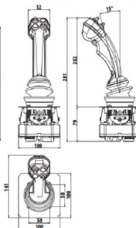
Med ergonomisk håndtag
