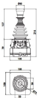
Med standard knop og poentiometre
