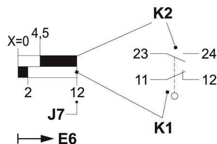
Kredsløbsdiagram
