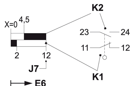
Kredsløbsdiagram
